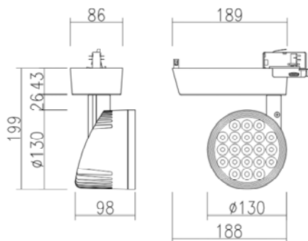
Technische Zeichnung
